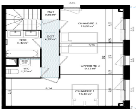
ÉTAGE R+2
